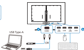
USB A-C
