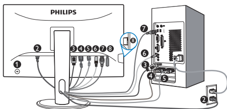
DVI (optional)
