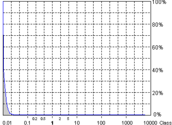
Flicker Emission - IEC 61000-3-3 , EN 61000-3-3 , (EN60555-3)
