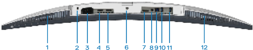
Vista inferior sin el pedestal del monitor
