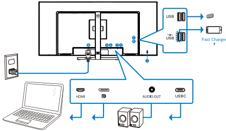
USB C-C
