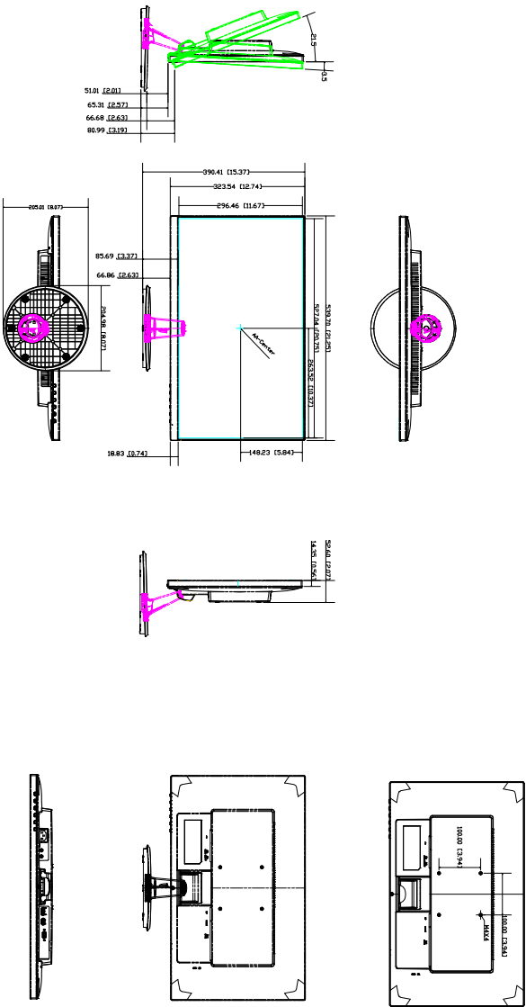
ASUS VA24DQ Outline Dimension
