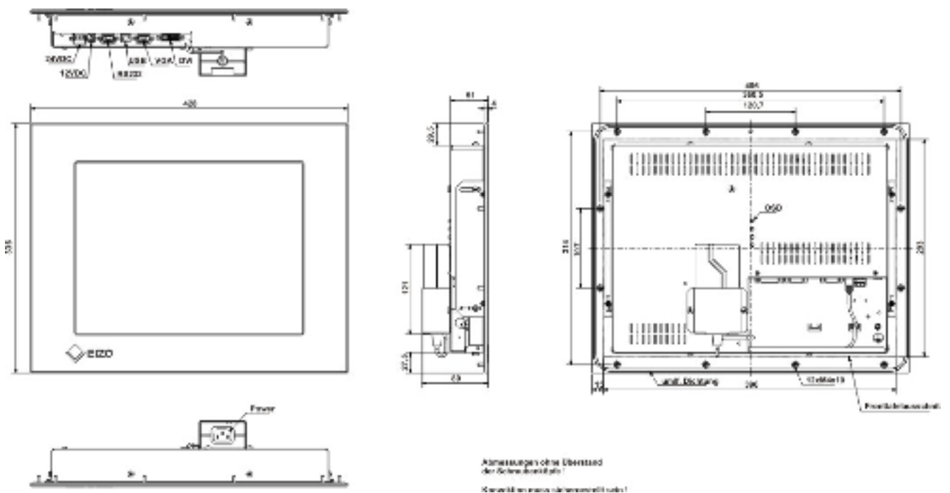
Abb. 1: Abmessungen des DV1508-002 (mit AC-Spannungsversorgung)
