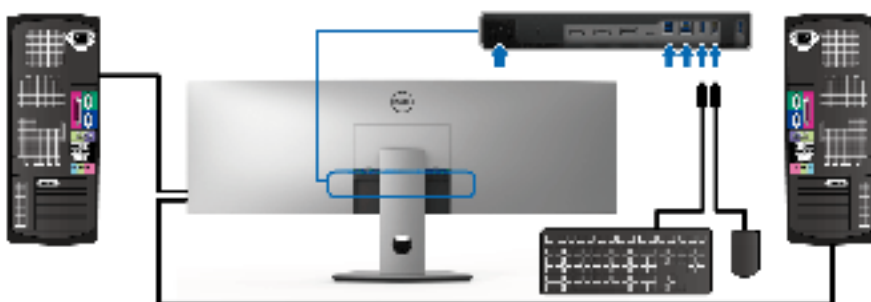
b. Conexión de dos ordenadores
