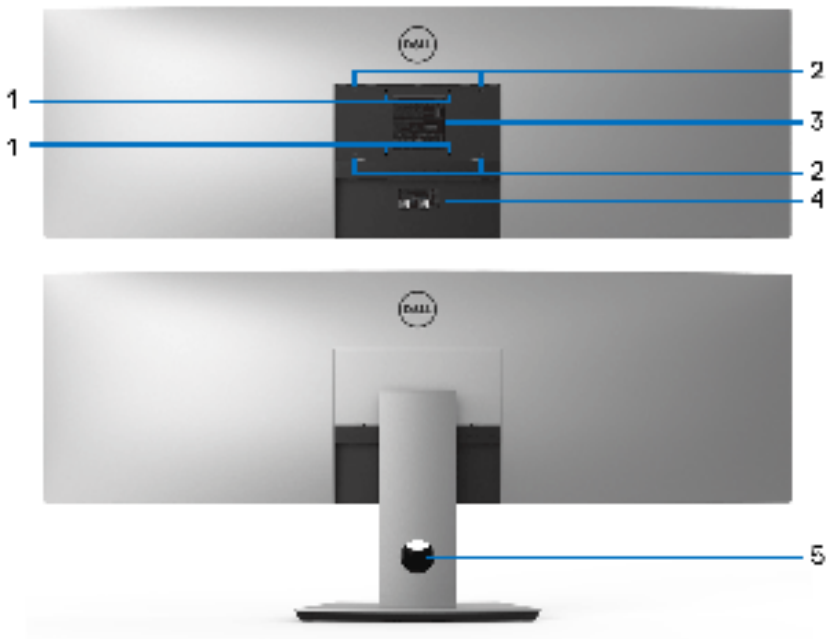
Vista trasera sin y con soporte de monitor
