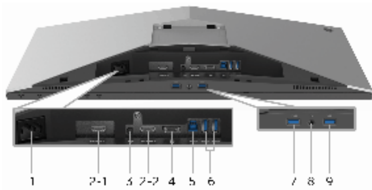
Vista trasera e inferior sin el soporte del monitor
